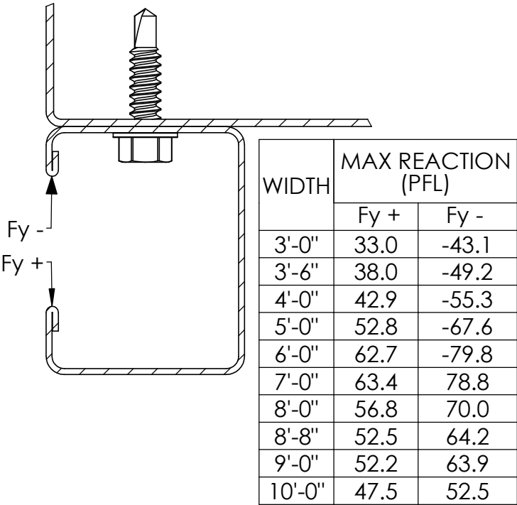
DOOR GUIDE FORCE
